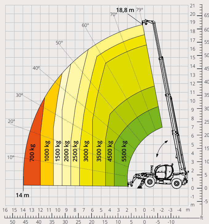
Diagramma portate con GANCIO 6.000 kg ATT-05-001
