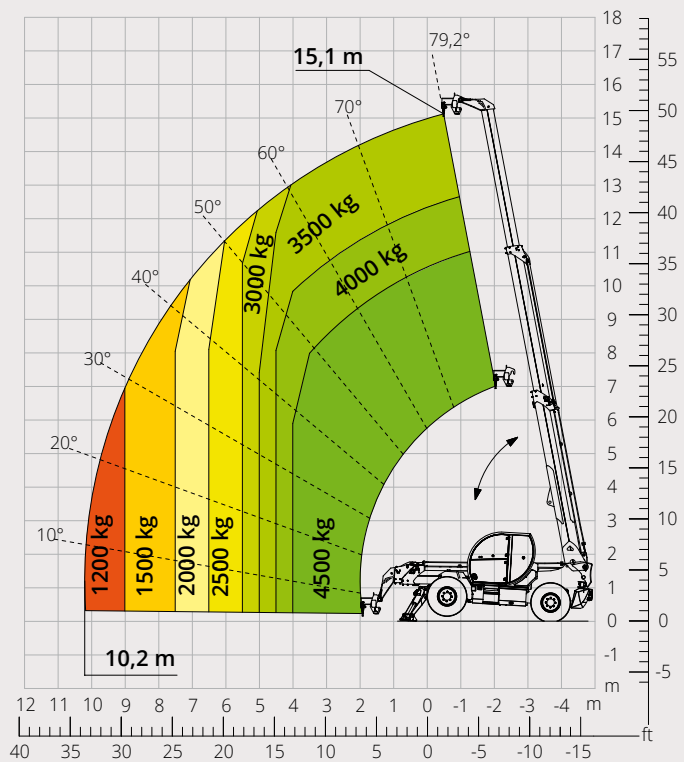
Diagramma portate con GANCIO 5.000 kg ATT-05-014
